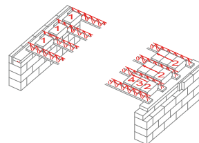
Postup ukladania stropných vložiek
