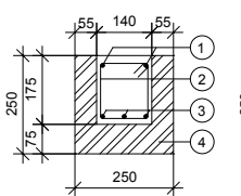
Preklad š. 250 mm
