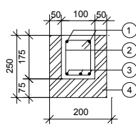
Preklad š. 200 mm
