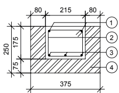
Preklad š. 375 mm
