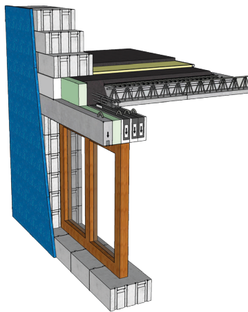
Vizualizácia skladby nosných a nenosných prekladov pri hrúbke steny 500 mm
