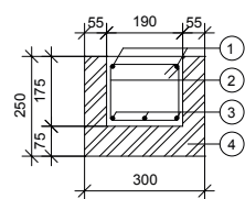
Preklad š. 300 mm
